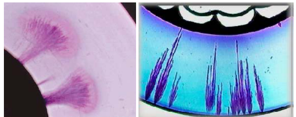
شکل ۲: رشد درختان آبی از طریق نیمه هادی خارجی ( سمت راست ) و نیمه هادی داخلی ( سمت چپ )
