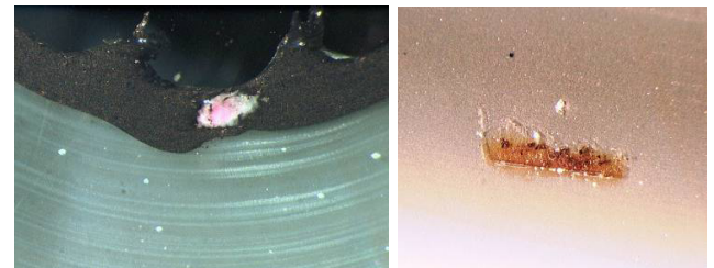
شکل ۶: عیوب نوعی دیده شده در کابل های با عایق اکستروود شده
